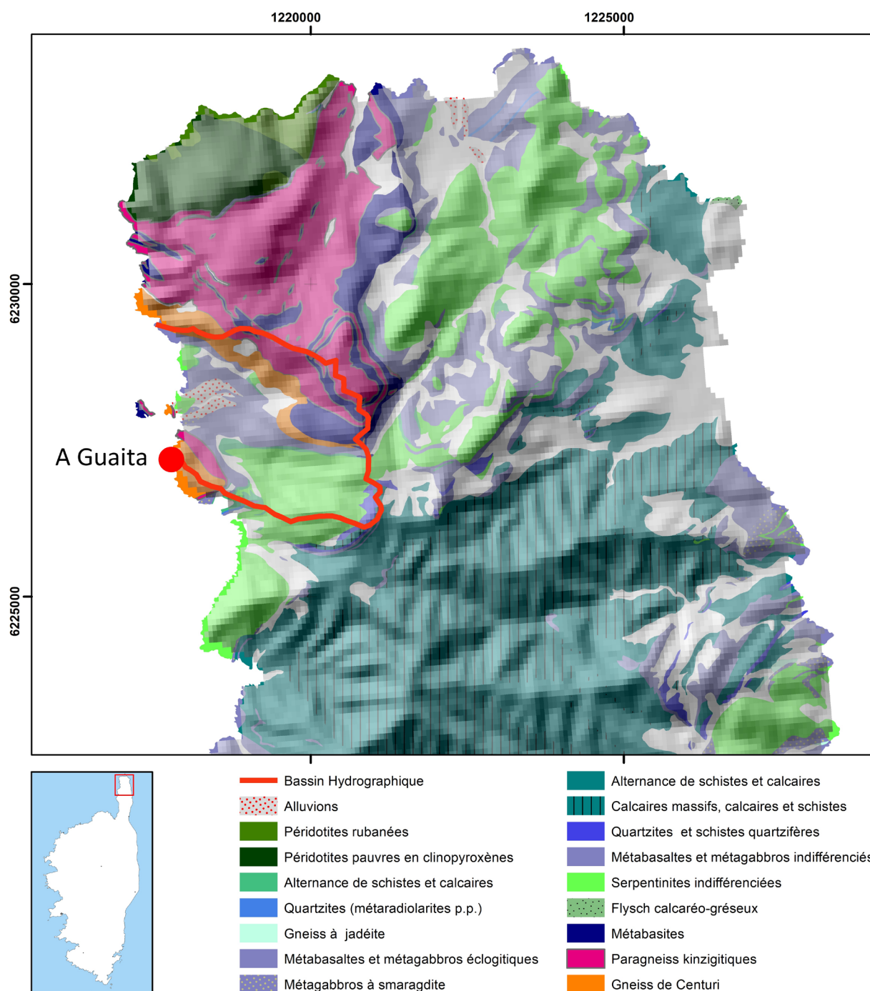
Fig. 2 – Carte lithologique simplifiée du Nord du Cap Corse (fond de carte : BRGM, carte géologique 1/50 000, Bd Charm-50, 2020 ; topographie – USGS SRTM 1- avec elevation data) (DAO : G. Boschian).
