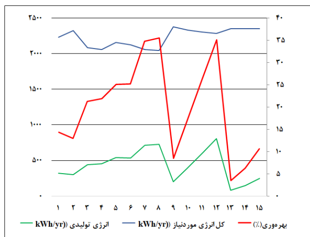
شکل ۵ میزان بازدهی انرژی نمونه‌های شبیه‌سازی‌شده
