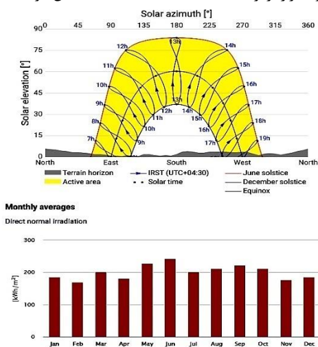
شکل ۴ تابش خورشیدی شهر شیراز [۶۴]
