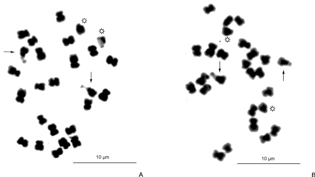
Fig. 1.- A-B: metafases mitóticas ( 2n = 26 ) de Pithecellobium dulce . Las flechas señalan a los cromosomas satelitados. Los asteriscos resaltan a los cromosomas subtelocéntricos.
